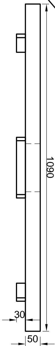
Sniðmynd
