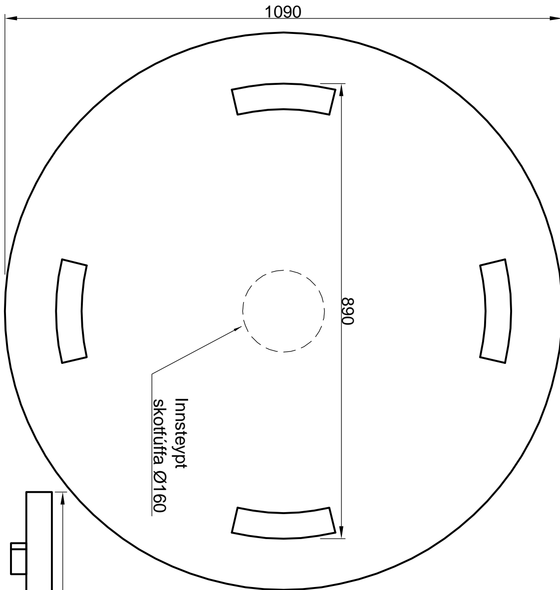
Grunnmynd, botn
